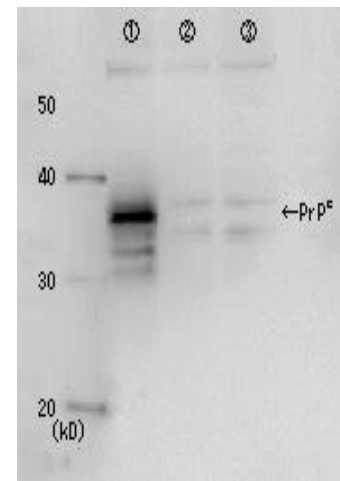
図1 抗プリオン蛋白質抗体(2C5-5)のウェスタンブロッティング (2,000倍希釈で使用) ①プリオン蛋白質過剰発現 RK13 細胞抽出液 ②コントロールベクター導入 RK13 細胞抽出液 ③RK13 細胞抽出液
